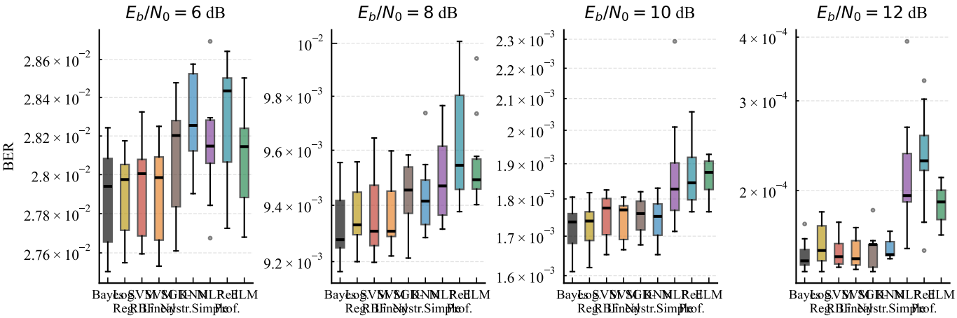
Distribución de BER por clasificador — E_b/N_0 clave
